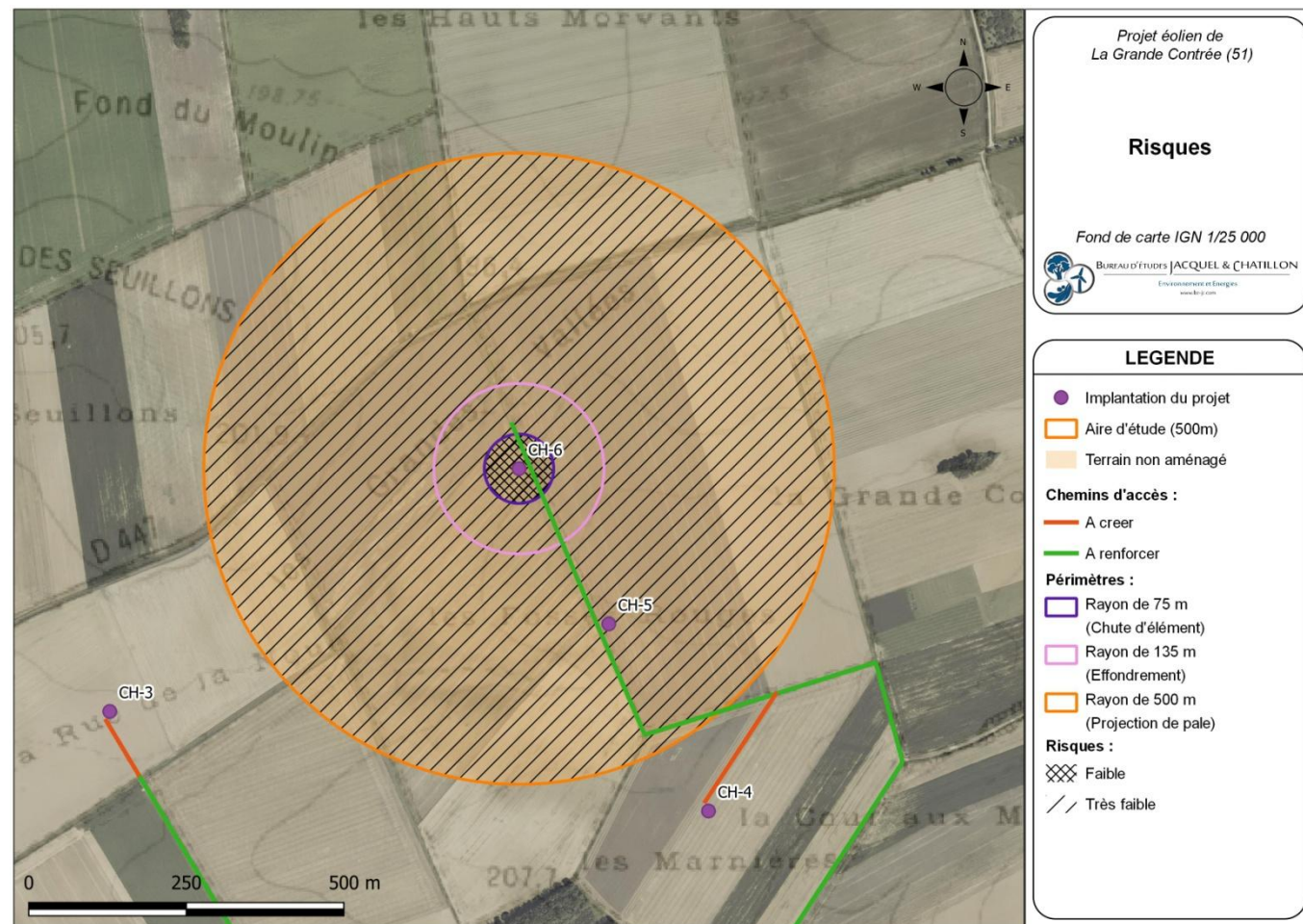
Carte 27 : Éolienne CH-6 – Risques liés à l'effondrement de l'éolienne, à la chute d'élément de l'éolienne, et à la projection de pale ou de fragment de pale (Source : BE Jacquel et Chatillon)
