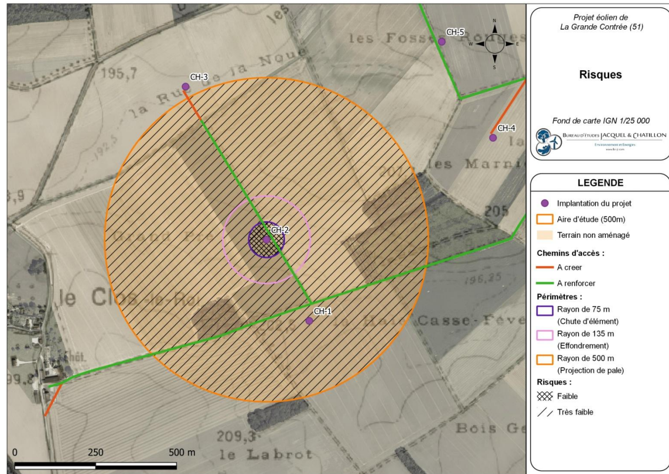
Carte 19 : Éolienne CH-2 – Risques liés à l'effondrement de l'éolienne, à la chute d'élément de l'éolienne, et à la projection de pale ou de fragment de pale (Source : BE Jacquel et Chatillon)
