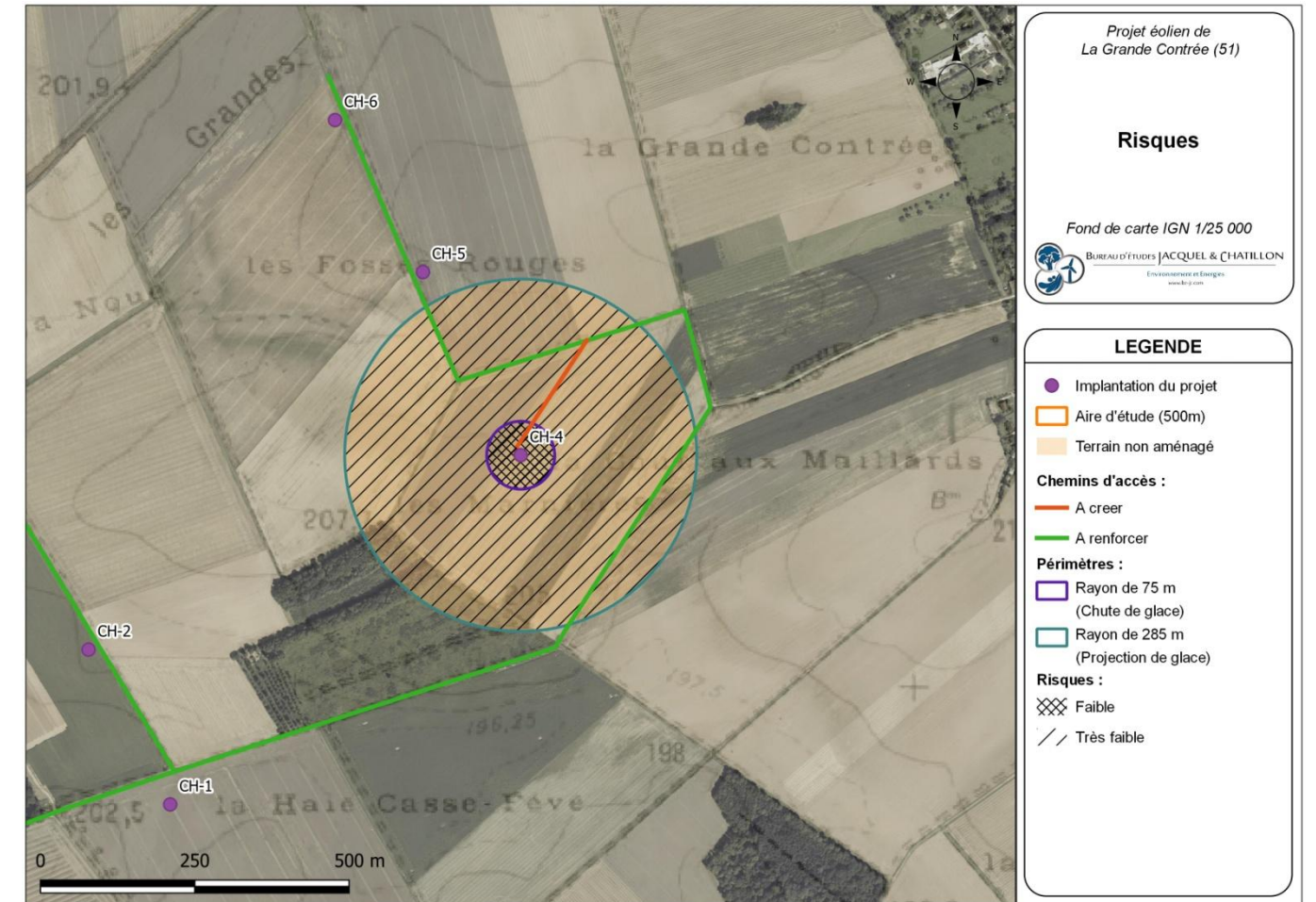
Carte 24 : Éolienne CH-4 – Risques liés à la chute et à la projection de glace (Source : BE Jacquel et Chatillon)
