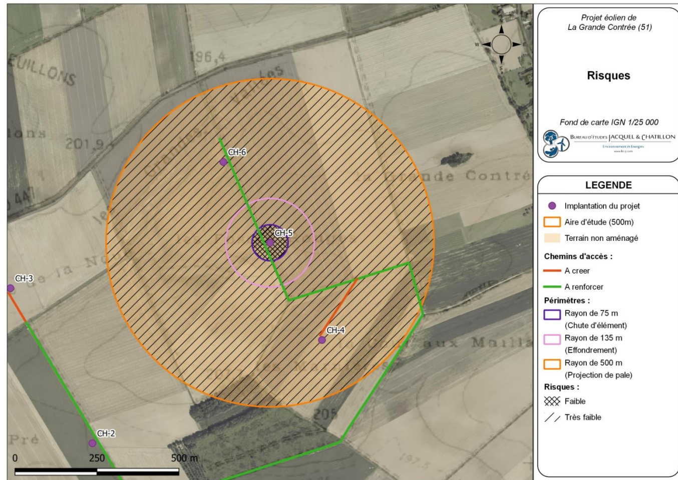
Carte 25 : Éolienne CH-5 – Risques liés à l'effondrement de l'éolienne, à la chute d'élément de l'éolienne, et à la projection de pale ou de fragment de pale (Source : BE Jacquiel et Chatillon)
