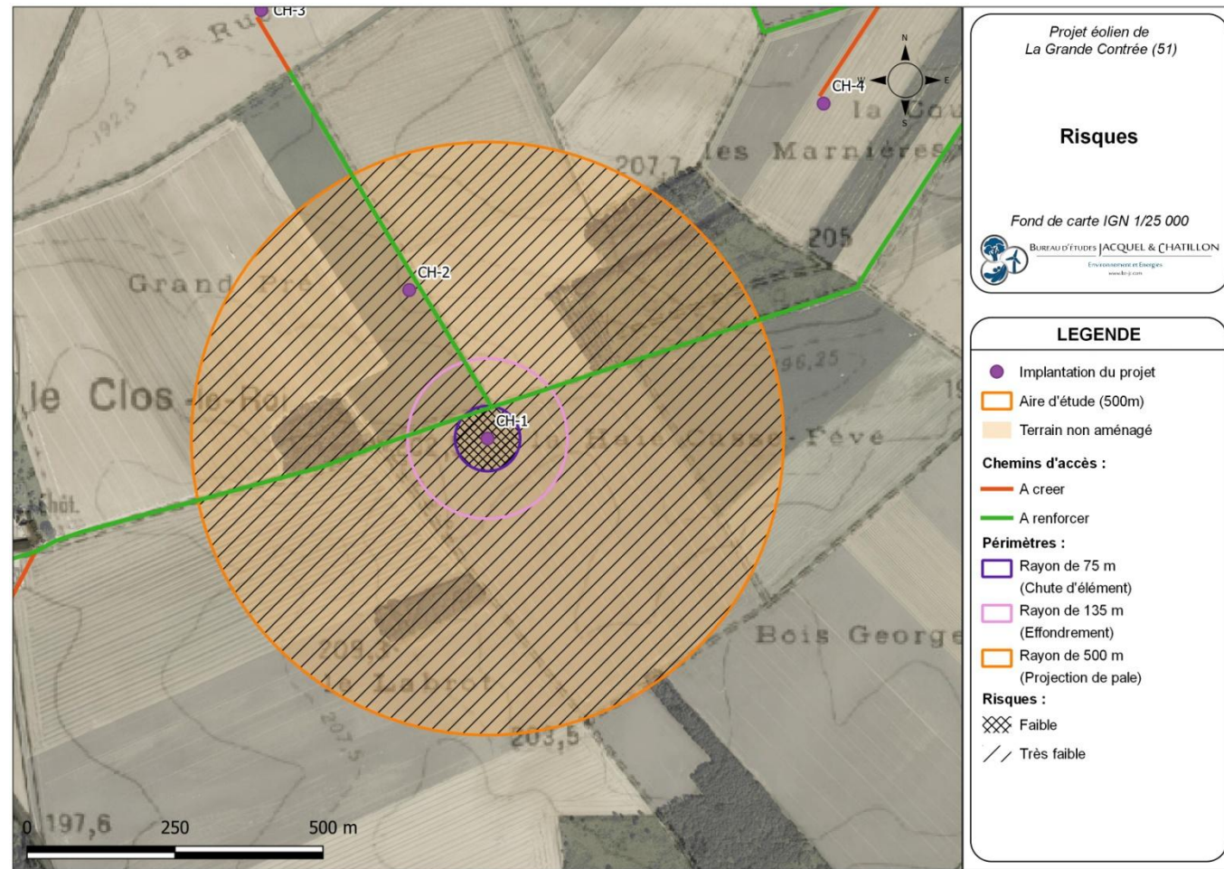
Carte 17 : Éolienne CH-1 – Risques liés à l'effondrement de l'éolienne, à la chute d'élément de l'éolienne, et à la projection de pale ou de fragment de pale (Source : BE Jacquel et Chatillon)
