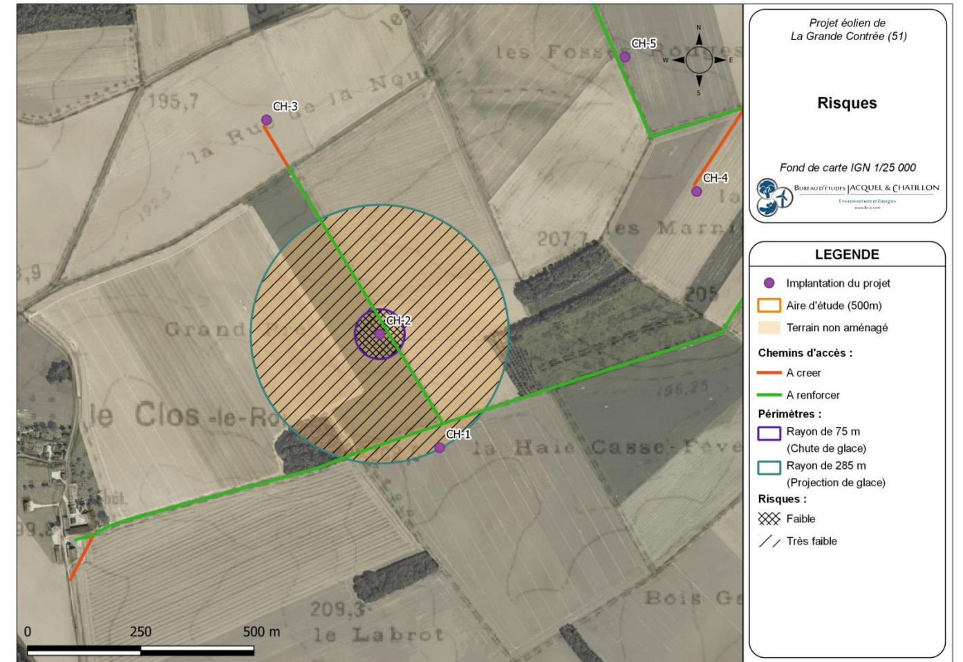
Carte 20 : Éolienne CH-2 – Risques liés à la chute et à la projection de glace (Source : BE Jacquel et Chatillon)
