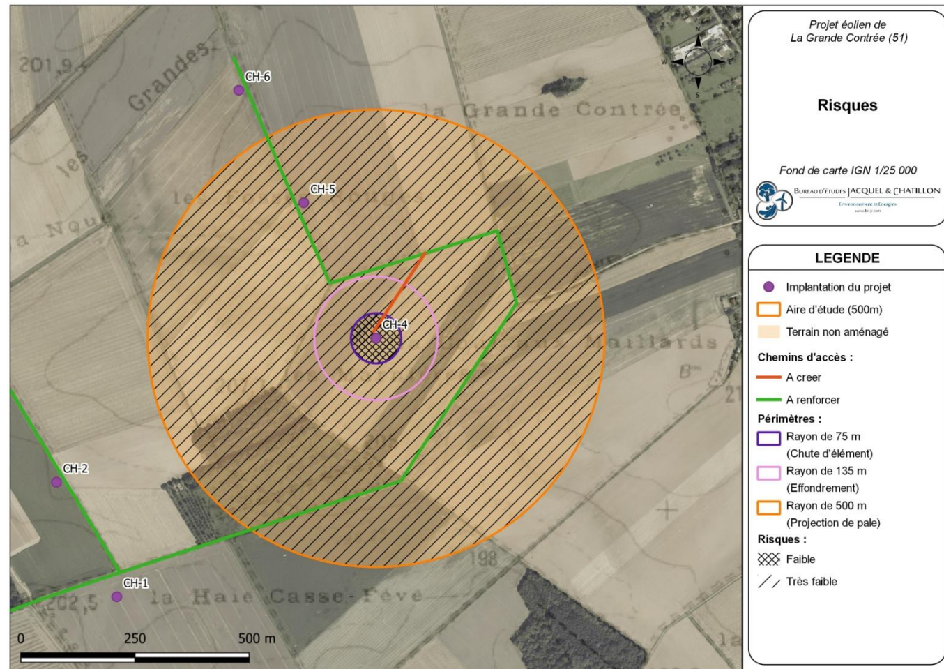
Carte 23 : Éolienne CH-4 – Risques liés à l'effondrement de l'éolienne, à la chute d'élément de l'éolienne, et à la projection de pale ou de fragment de pale (Source : BE Jacquel et Chatillon)
