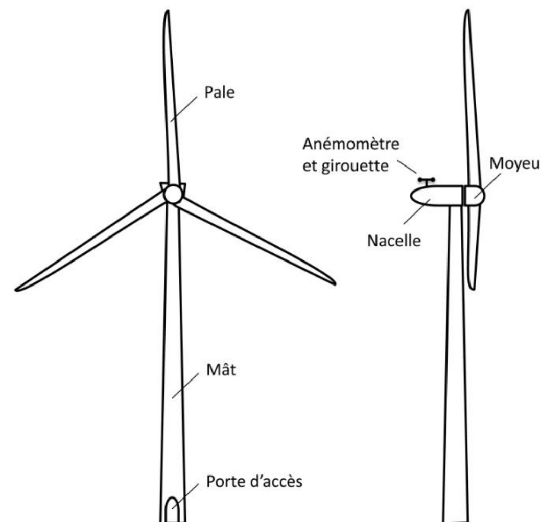
Figure 1 : Schéma simplifié d'un aérogénérateur (Source : INERIS)
