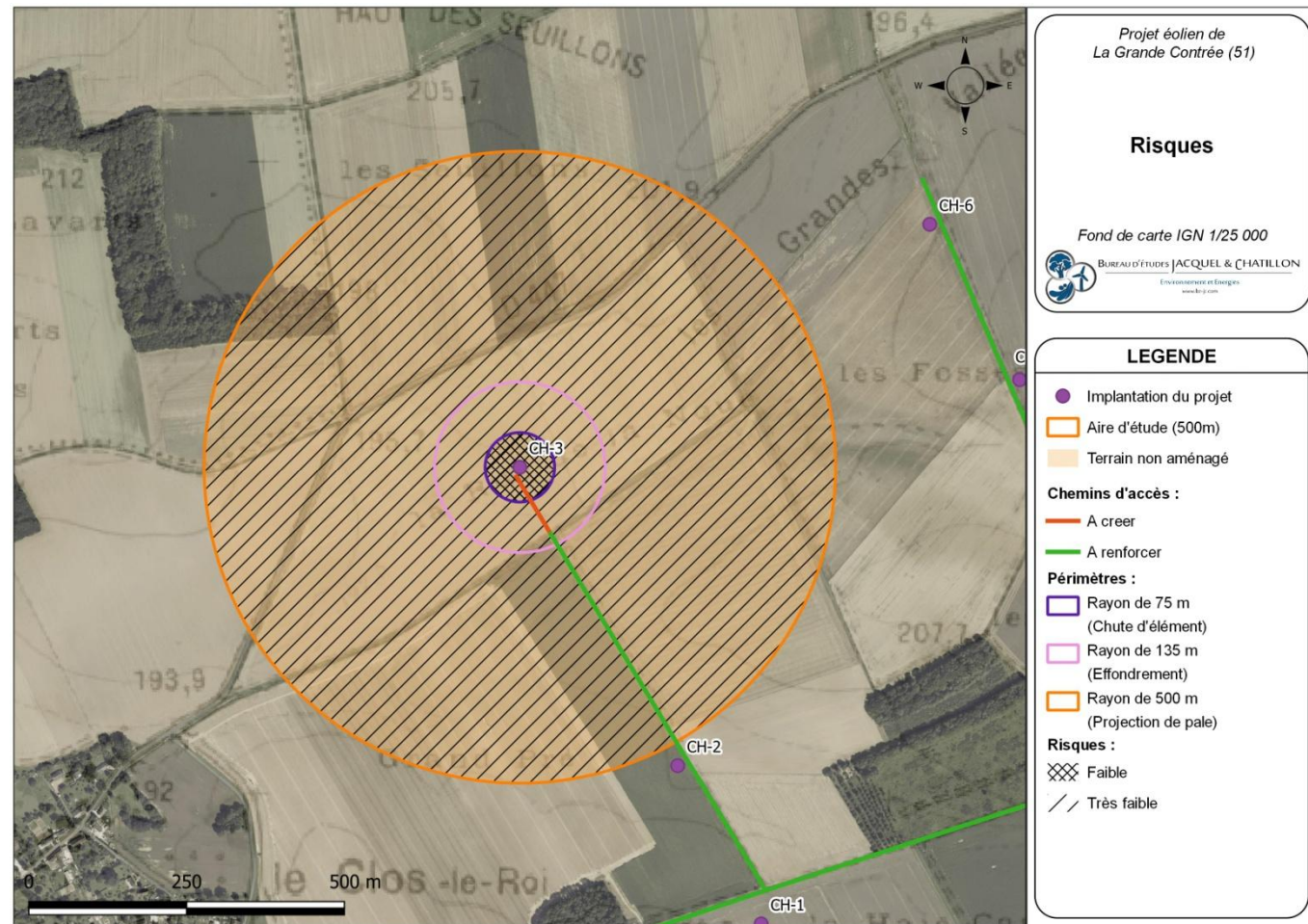
Carte 21 : Éolienne CH-3 – Risques liés à l'effondrement de l'éolienne, à la chute d'élément de l'éolienne, et à la projection de pale ou de fragment de pale (Source : BE Jacquiel et Chatillon)
