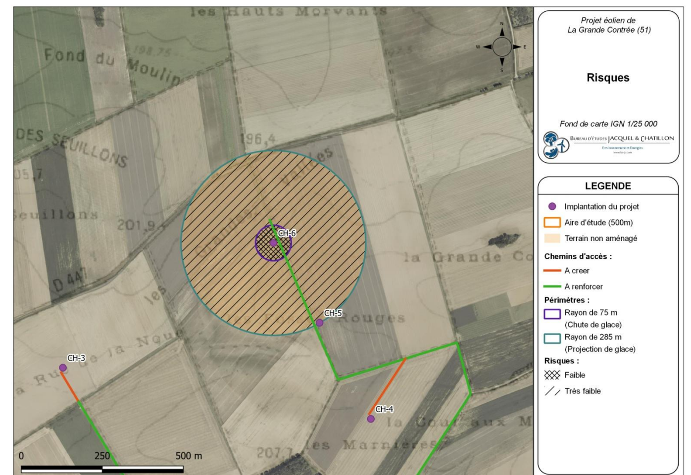
Carte 28 : Éolienne CH-6 – Risques liés à la chute et à la projection de glace (Source : BE Jacquel et Chatillon)
